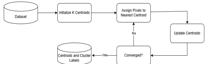
Gambar 4. Tahapan ekstraksi fitur menggunakan algoritma K-Means .
