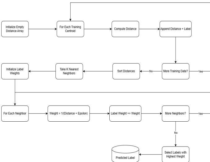
Gambar 6. Tahapan klasifikasi menggunakan algoritma modified KNN.
