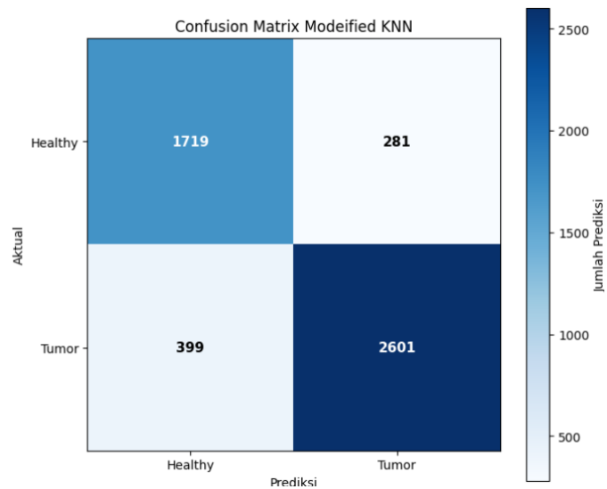
Gambar 11. Hasil Confusion Matrix Modified KNN pada dataset lain.
